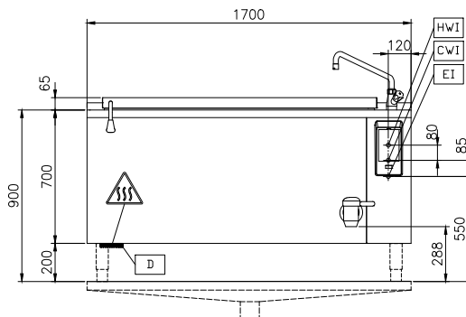
Zij aanzicht
